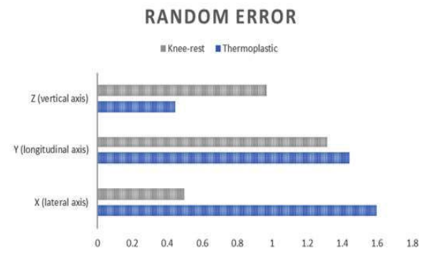
Fig. 2: Random error
